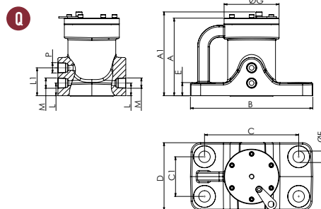
ESPECIFICACIONES DIMENSIONALES
