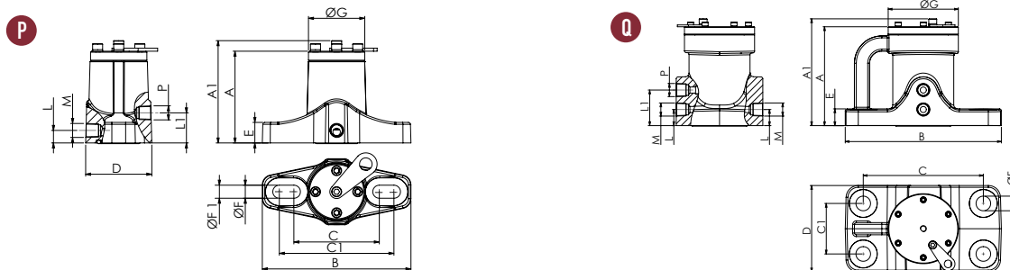
ESPECIFICACIONES DIMENSIONALES
