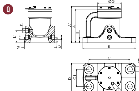
SPÉCIFICATIONS DIMENSIONNELLES
