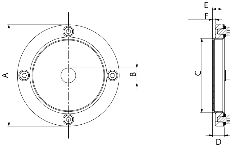
SPÉCIFICATIONS DIMENSIONNELLES
