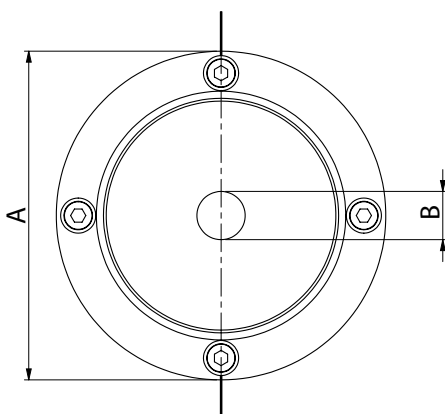
ESPECIFICAÇÕES DIMENSIONAIS
