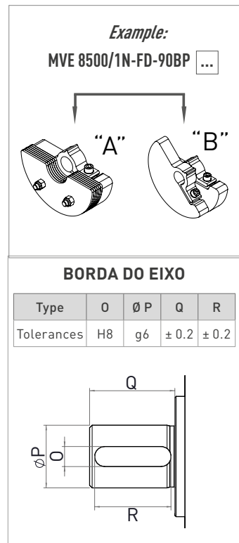
Chave paralela com ponta redonda DIN 6885 A
