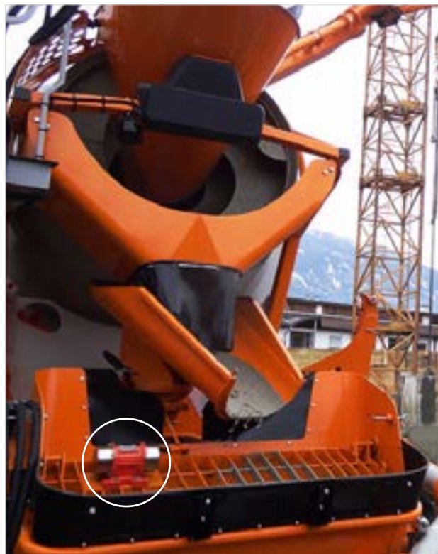
MVE-DC (elektryczny wibrator) - Pompa do betonu
