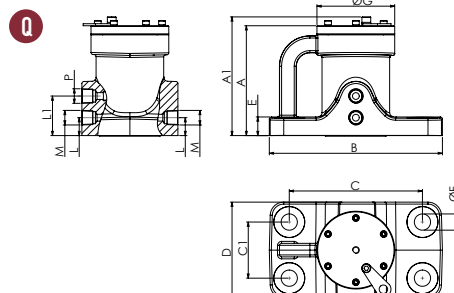
SPECYFIKACJE WYMIAROWE
